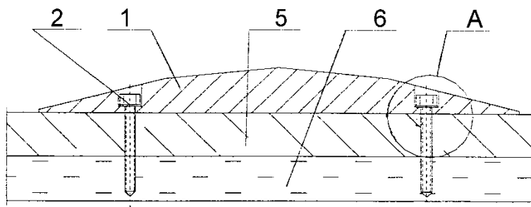
Szczegół A
