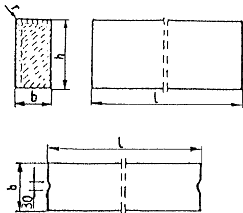
Rys. 1. Wymiarowanie krawężników
