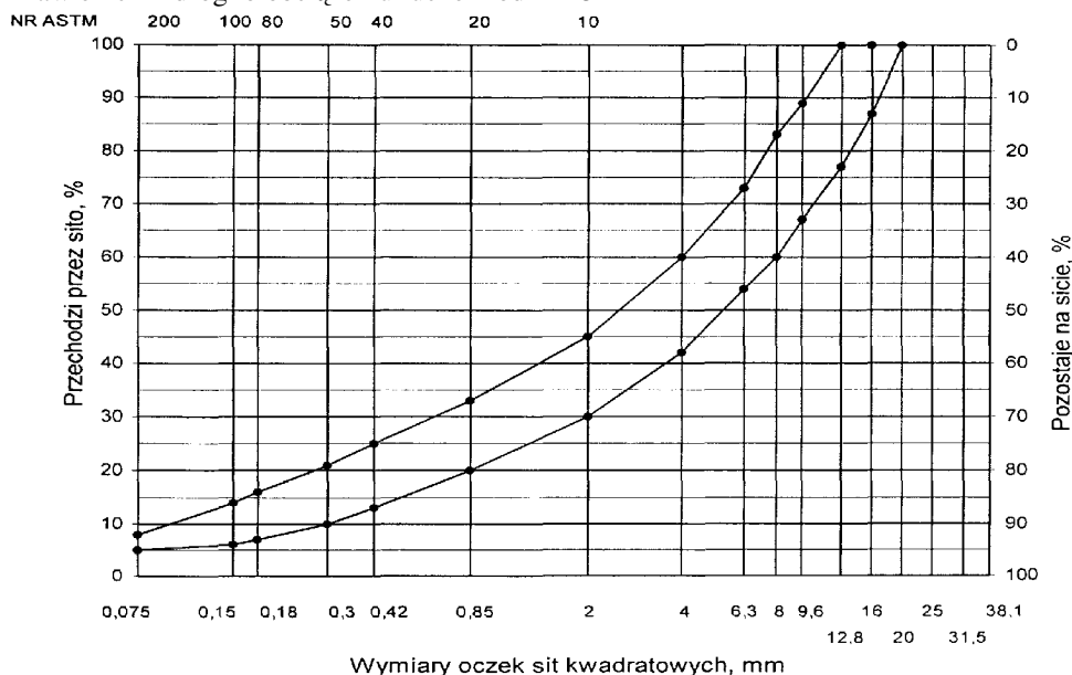
Rys. 1. Krzywe graniczne uziarnienia mieszanki mineralnej BA od 0 do 25 mm do warstwy wiążącej, nawierzchni drogi o obciążeniu ruchem od KR 3
