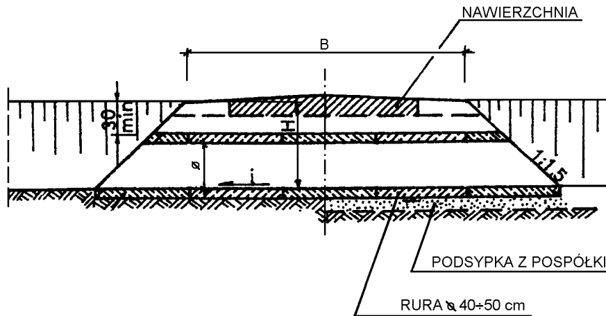
Rys. 3.2. Przekrój podłużny przepustu z rury polietylowej średnicy 40÷50 cm pod zjazdem
