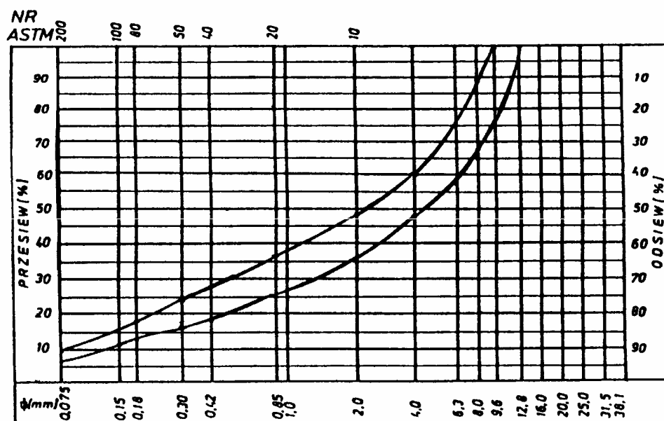
Rys. 7. Krzywe graniczne uziarnienia mieszanki mineralnej 0-12,8 mm do warstwy ściernicowej z betonu asfaltowego dla KR 3-6
