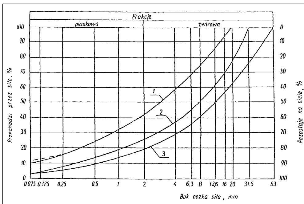
Rysunek 1. Pole dobrego uziarnienia kruszyw przeznaczonych na podbudowy wykonywane metodą
