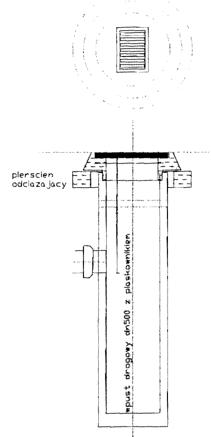
Typowy wpust drogowy na studzience betonowej dn500 podz. 1:20
