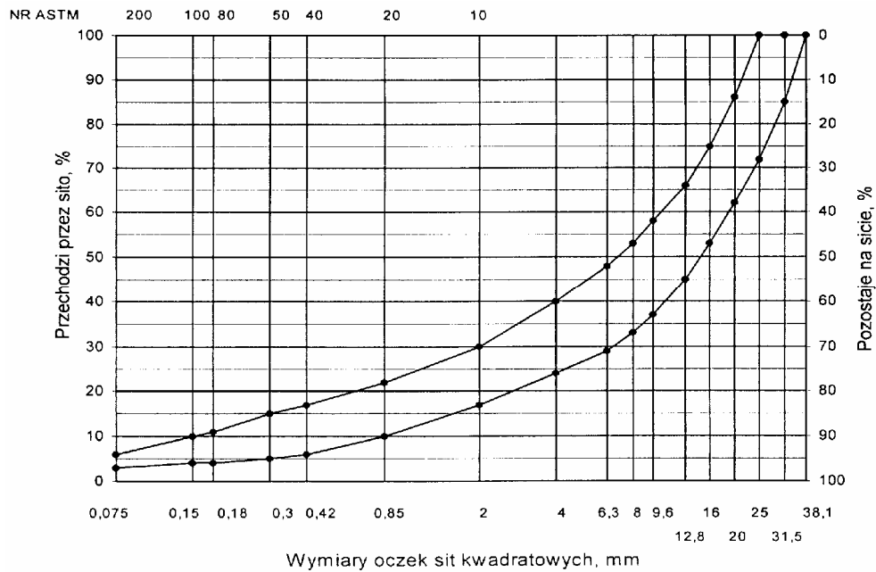
Tablica 2. Rzędne krzywych granicznych uziarnienia mieszank mineralnych do podbudowy z betonu asfaltowego oraz orientacyjne zawartości asfaltu
