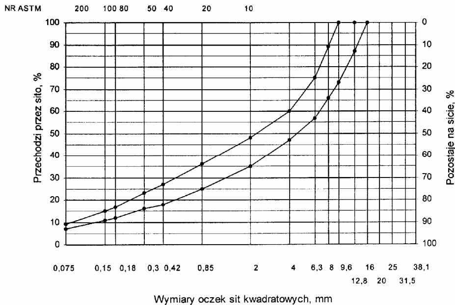
Rys. 4. Krzywe graniczne uziarnienia mieszanki mineralnej BA od 0 do 12,8 mm do warstwy ścieralnej na powierzchni drogi o obciążeniu ruchem od KR3 do KR6
