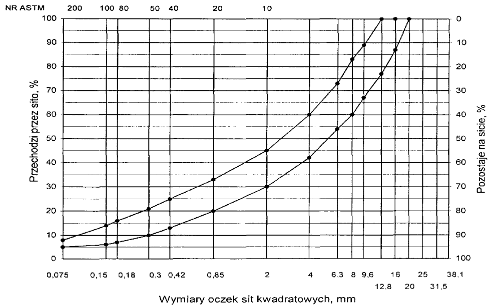
Rys. 3. Krzywe graniczne uziarnienia mieszanki mineralnej BA od 0 do 16 mm do warstwy wyrównawczej nawierzchni drogi o obciążeniu ruchem od KR3 do KR6
