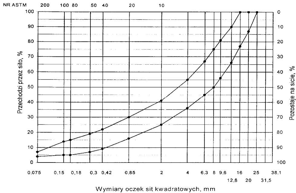
Rys. 2. Krzywe graniczne uziarnienia mieszanki mineralnej BA od 0 do 20 mm do warstwy wiążącej, wyrównawczej i wzmacniającej nawierzchni drogi o obciążeniu ruchem od KR3 do KR6
