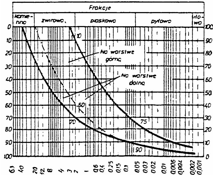
Rysunek 2. Obszar uziarnienia optymalnych mieszank gliniasto-żwirowych
