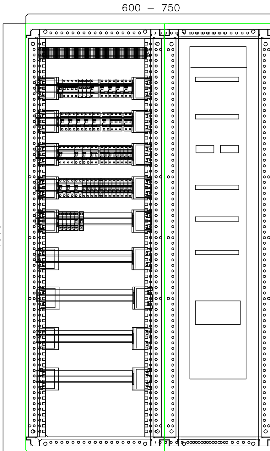
głębokość rozdzielnic 245-270 mm dla układu UFC107E-65-06-B16
