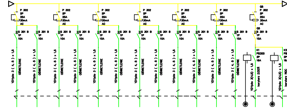
obwody oświetlenia, 2 piętro - SEGMENT B
