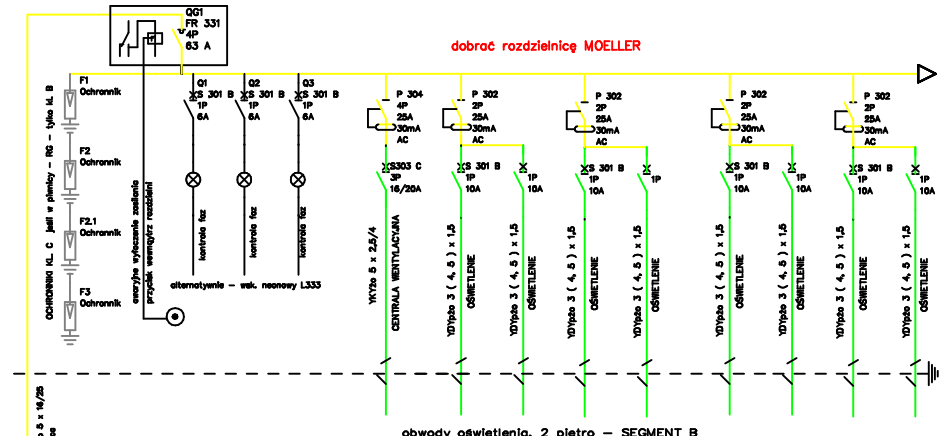
obwody oświetlenia, 2 piętro - SEGMENT B
