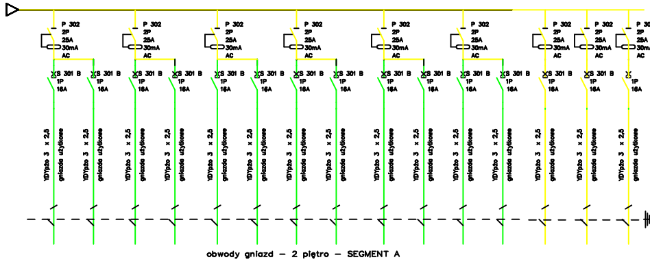
obwody gniazd - 2 piętro - SEGMENT A
