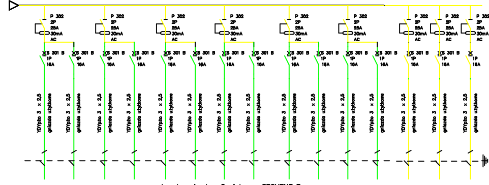
obwody gniazd - 2 piętro - SEGMENT B
